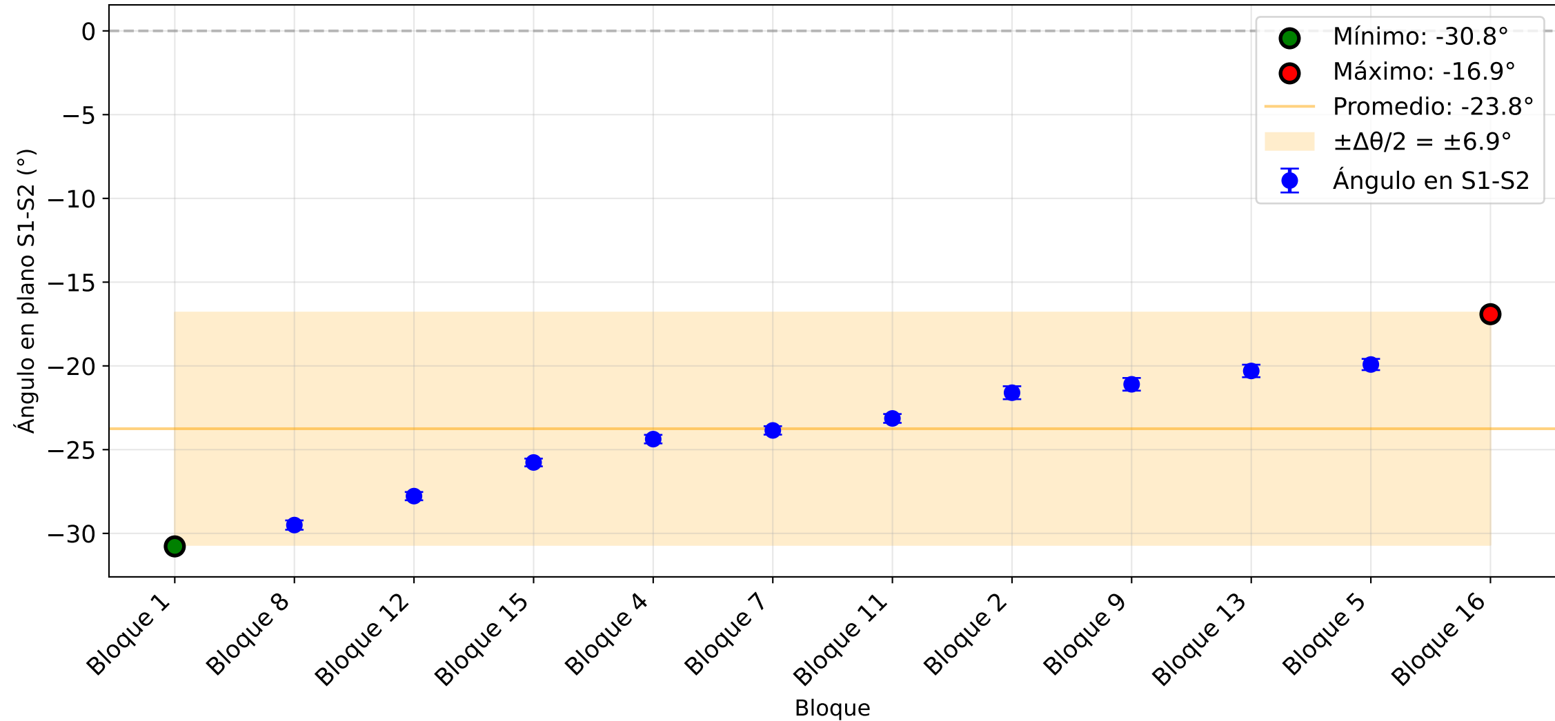
Dispersión angular en S1-S2: \Delta\theta = 13.9^\circ \pm 0.4^\circ
